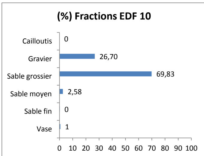
Figure 4634 : Analyse granulométrique
