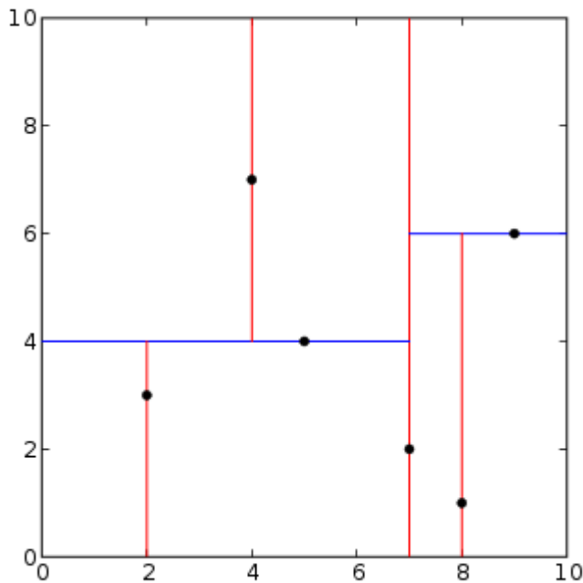
Figure 9 : Représentation schématique de la décomposition d'un jeu de données par un K-d tree
