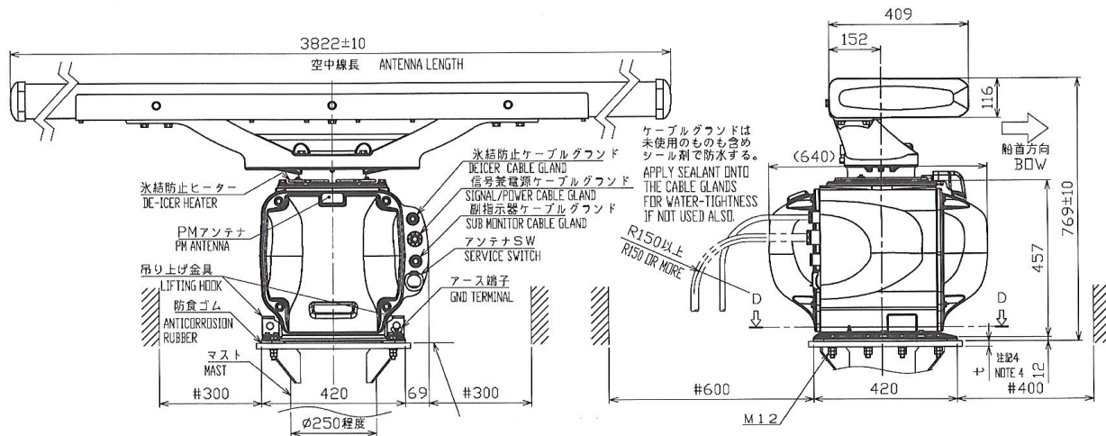
Figure 2 : Dimensions du radar en bande S
