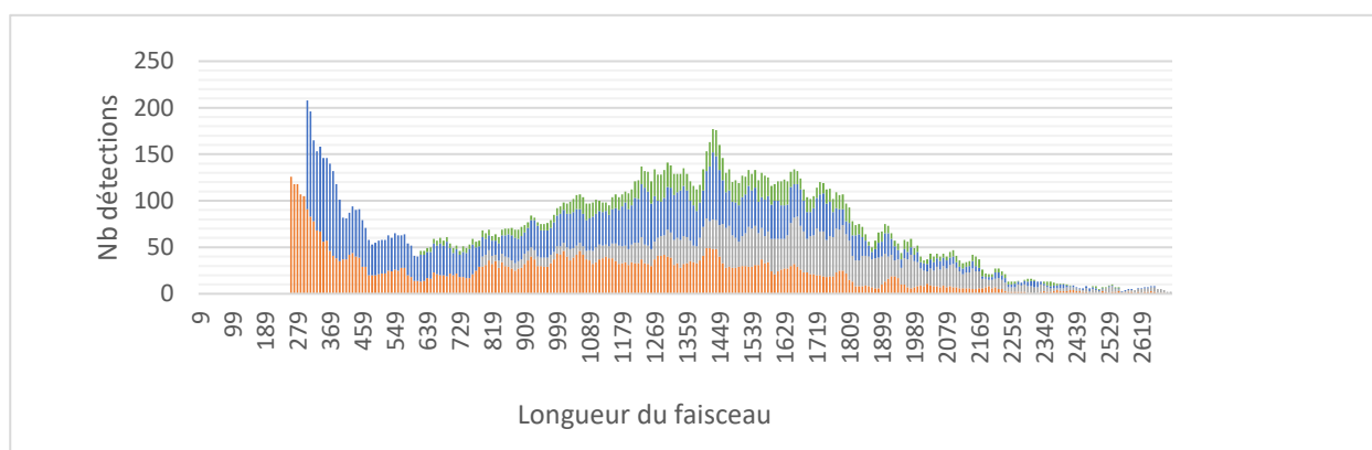
Figure 14 : Evolution de la détectabilité des cibles en fonction de la distance
