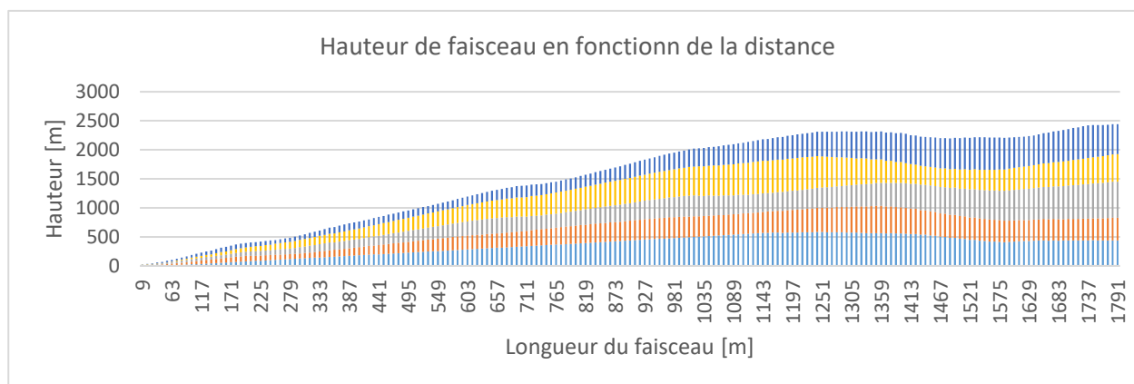
Figure 13 : Evolution de la hauteur du faisceau en fonction de la distance
