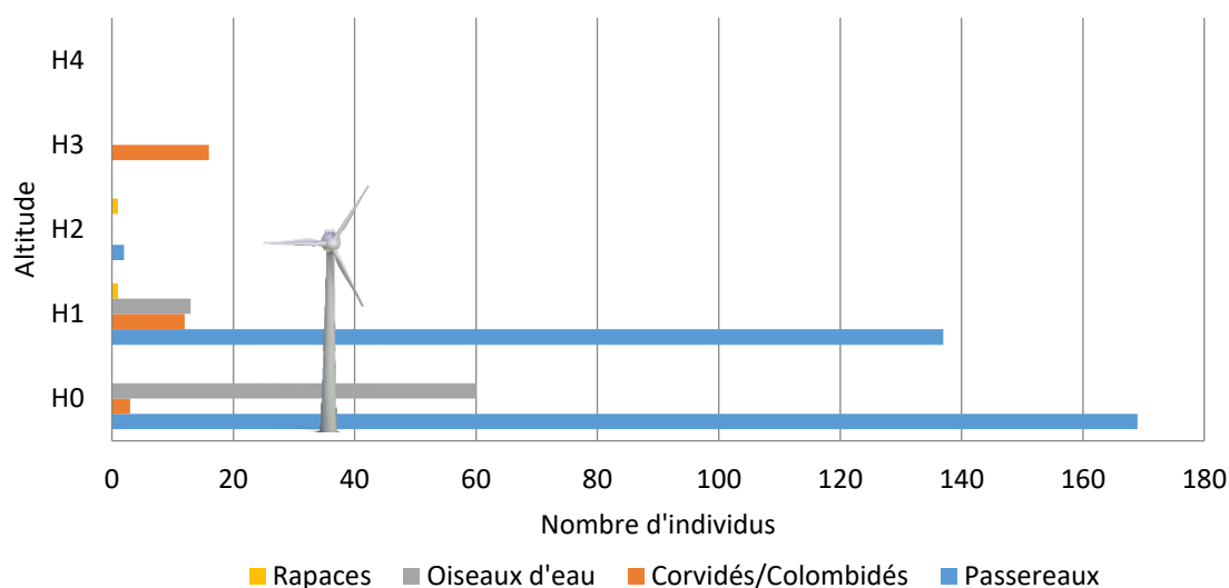
Figure 21 : Hauteurs de vol pendant la migration postnuptiale au Cap Fréhel - H0 = repos, H1 = en-dessous des pales (0-130m), H2 = à hauteur de pales (130-210m), H3 = au-dessus des pales (210-250m) et H4 = bien au-dessus des pales (>250m)
