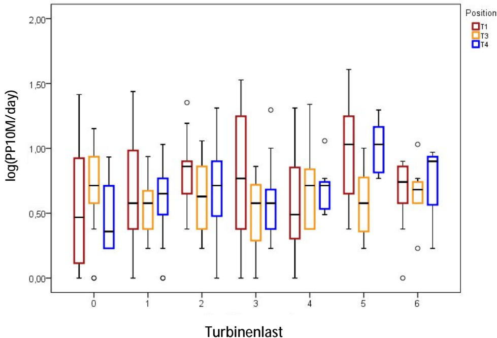
Fig. 6-7: Schweinswal-Detektionsraten PP10M/day im Nahbereich des Windparks alpha ventus (POD-Stationscluster ‚Impact Area‘) bei unterschiedlicher Turbinenlast (Volllast = 6).
