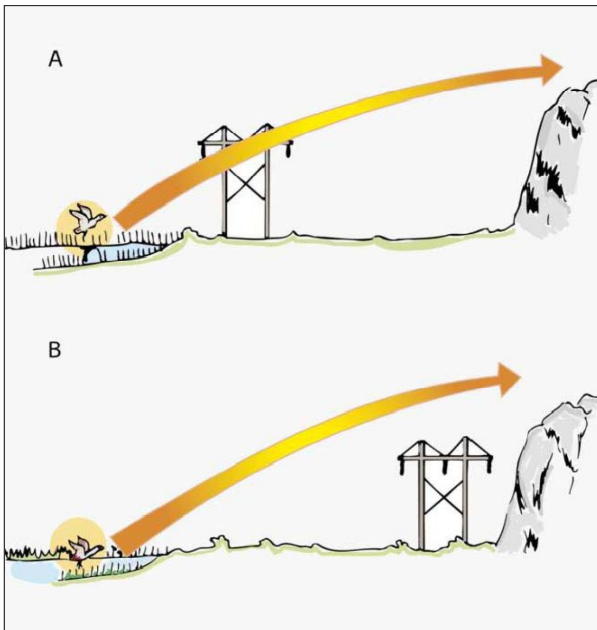
Figur 18. Ved å legge kraftledninger nært inntil bergvegger og skreenter kan fuglene "tvinges" til å øke flygehøyden slik at kollisjon med linene unngås (etter Avery 1978).
