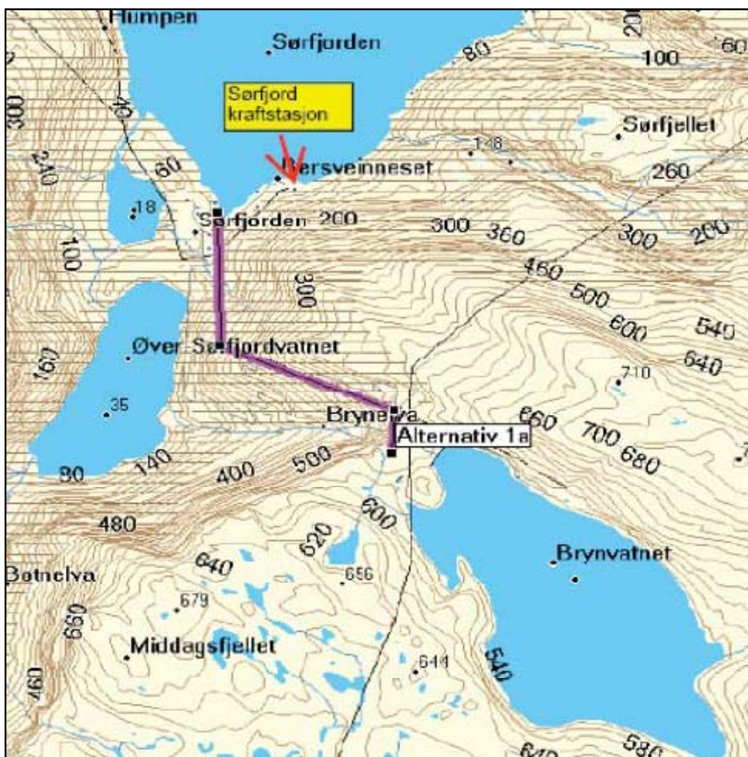
Figur 3. Det planlegges å rive eksisterende 22 kV linje som går fra Sørjorden og inn til det aktuelle tiltaksområdet. Traseen skal benyttes til bygging av ny 132 kV linje. Denne linjen tilknyttes eksisterende 132 kV linje (Sørjorden-Kjøpsvik) ved Sørjorden kraftstasjon.
