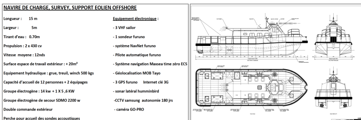
Figure 4 : Caractéristiques du Celtic Warrior
