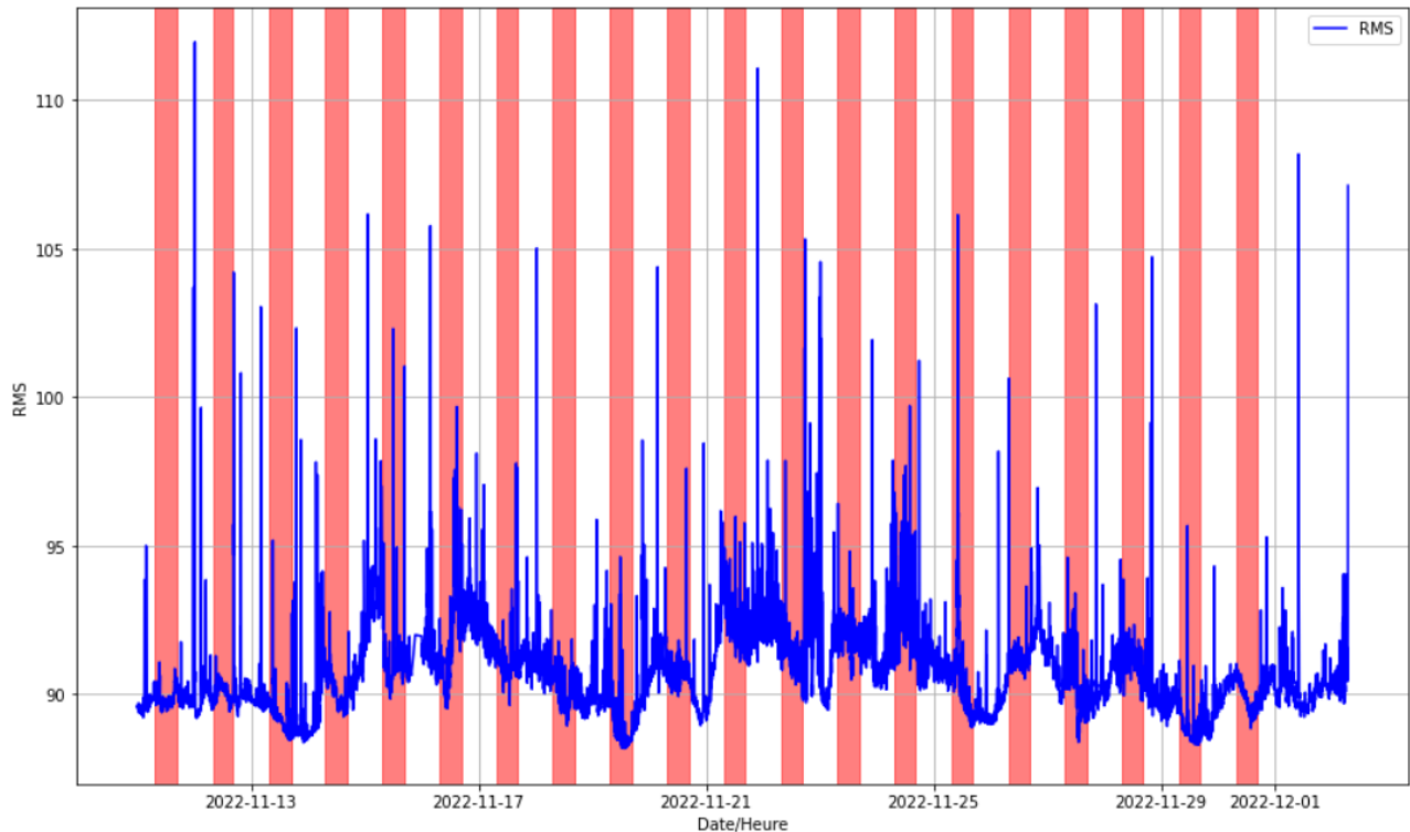
Figure 13 : Niveau de bruit sous-marin associé aux espèces benthiques (4 kHz à 20 kHz) mesuré en décibels (dB re \mu\text{Pa} ) en fonction du cycle nyctéméral (en orange les périodes de jour) du 11/11/2022 au 30/11/2022.
