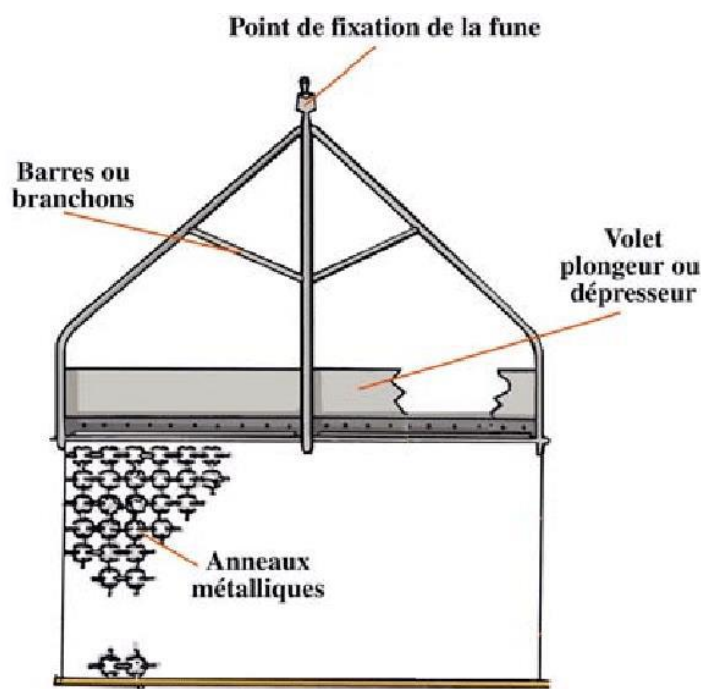
Figure 3: Schéma d'une drague classique (george, 2005)
