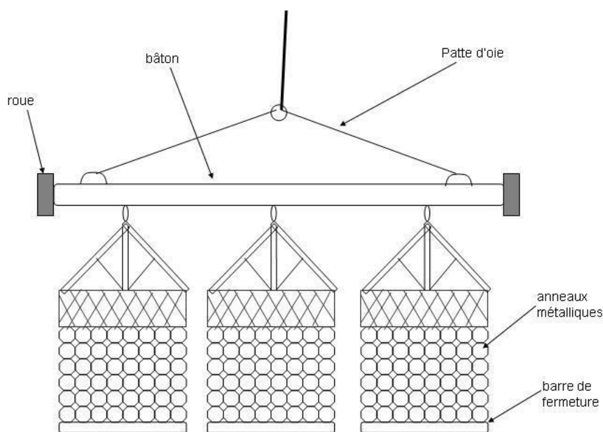
Figure 2: Schéma d'une drague anglaise (source : www.crpb.fr )
