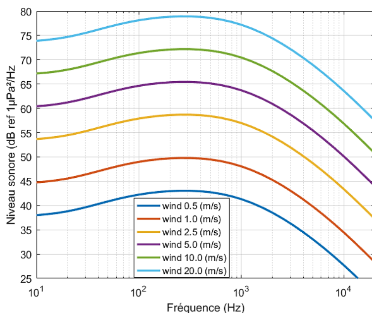
Figure 20 : Niveau sonore induit par le vent en fonction de la fréquence et de la vitesse.
