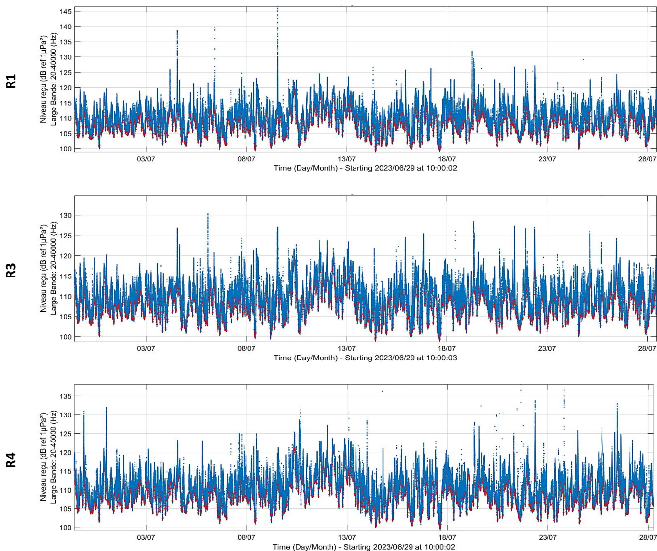
Figure 13 : Evolution des niveaux intégrés dans la bande [20Hz;40kHz] (entre 20 Hz et 40 kHz, exprimés en dB ref 1µPa 2 ) mesurés lors de la période été 2023.
