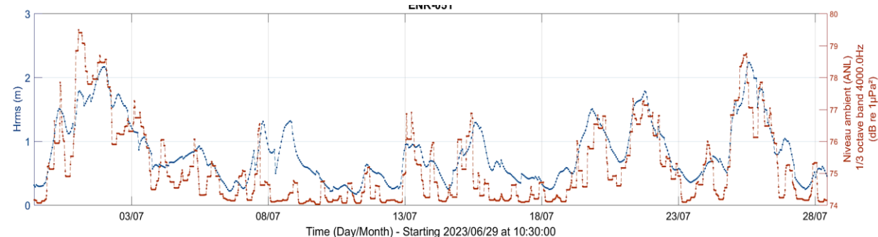
Figure 14 : Corrélation du bruit permanent (orange) avec les conditions météorologiques (bleu) dans la zone d'étude lors période été 2023.
