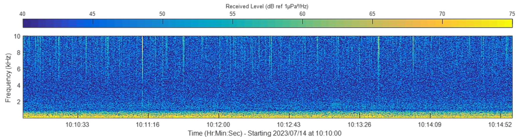
Figure 16 : Spectrogrammes d'événements acoustiques repérés lors de la période été 2023, à proximité de la station R4.
