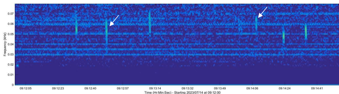
Figure 54 : « Downsweep chirp » émis par le Rorqual commun, Balaenoptera physalus , entre 65 Hz et 45 Hz à proximité de la station R3. Enregistrement du 14/07/2023 vers 09h12 UTC.
