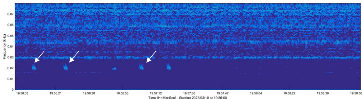
Figure 42 : Pulses émis en doublet par un Rorqual commun, Balaenoptera physalus , entre 27 Hz et 17 Hz (« 20-Hz signal ») à proximité de la station R1. Enregistrement du 10/03/2023 vers 19h56 UTC.
