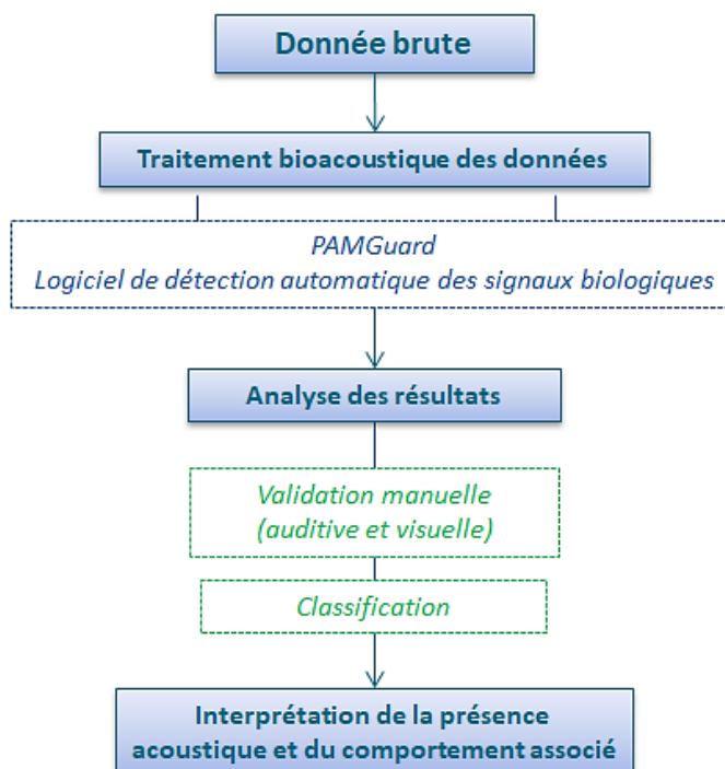
Figure 35 : Procédure générale appliquée à la donnée brute pour le traitement bioacoustique des enregistrements sonores.
