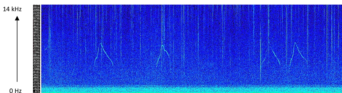
Figure 46 : Sifflements probablement émis par le Dauphin commun ( Delphinus delphis ) entre 7 et 15 kHz le 06/03/2023 vers 21h56 UTC au niveau de la station R3.
