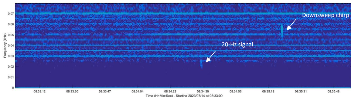
Figure 52 : Emission seul d'un « 20-Hz signal » entre 27 Hz et 17 Hz, ainsi que d'un « downsweep chirp » entre 60 Hz et 50 Hz par un Rorqual commun, Balaenoptera physalus , à proximité de la station R4. Enregistrement du 14/07/2023 vers 08h33 UTC.
