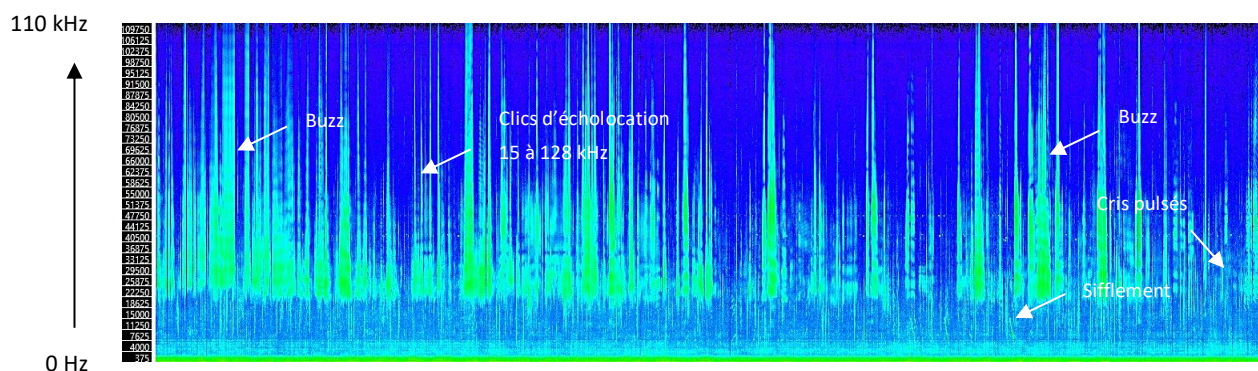
Figure 49 : Episode de chasse avec l'émission de trains de clics d'écholocation, buzz, cris pulsés et sifflements par les Delphinidés à proximité de la station R3. Enregistrement du 30/06/2023 vers 09h58 UTC.
