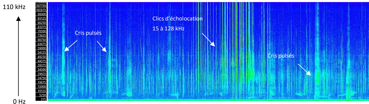
Figure 40 : Présence significative de cris pulsés émis par les Delphinidés évoquant une activité intense à proximité de la station R4. Enregistrement du 10/03/2023 vers 22h58 UTC.
