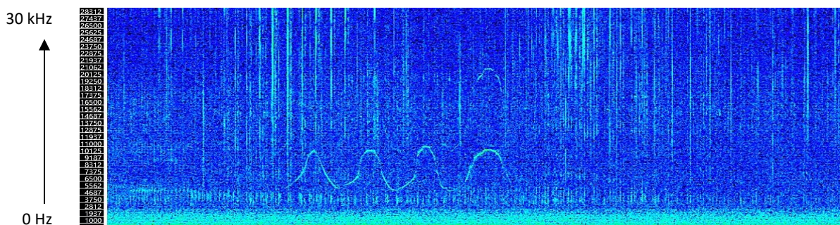
Figure 56 : Sifflements émis par le Grand Dauphin ( Tursiops truncatus ) entre 3 et 12 kHz le 30/06/2023 vers 07h32 UTC au niveau de la station R3.
