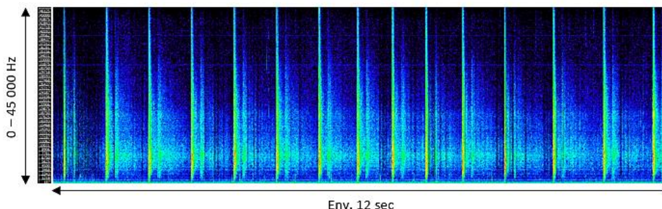
Figure 34 : Clics de Cachalot macrocéphale ( Physeter macrocephalus ) entre 2 et 30 kHz. Source : Quiet-Oceans.
