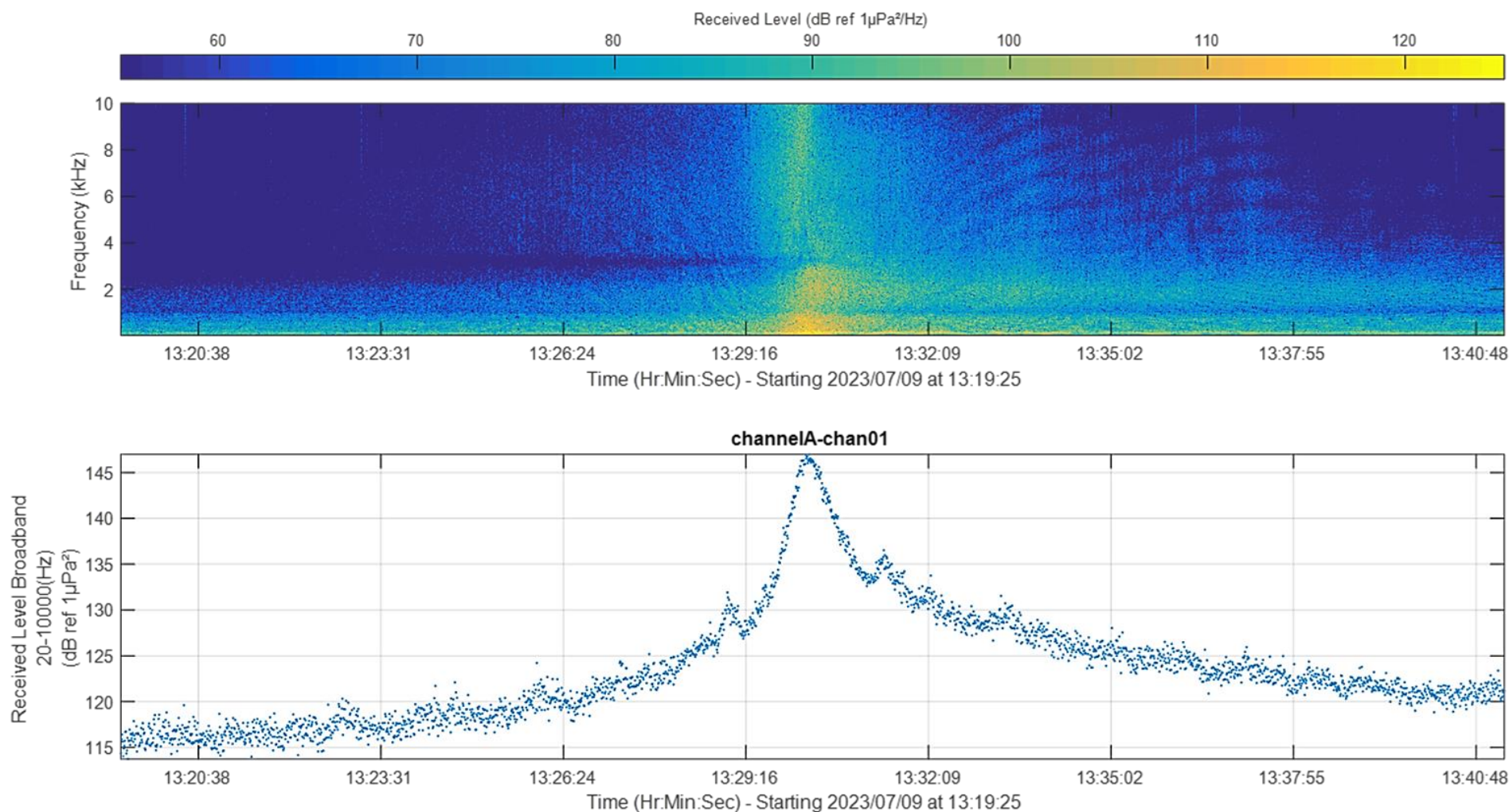
Figure 15 : En haut, spectrogramme du passage proche du navire cargo « GLEN » à proximité de la station R1, dans la journée du 09 Juillet 2023. En bas, niveau sonore associé à ce passage de navire (20Hz-10kHz) exprimé en dB ref 1 \mu\text{Pa}^2 .
