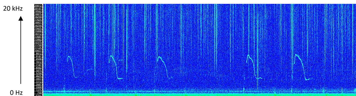
Figure 55 : Sifflements émis par le Grand Dauphin ( Tursiops truncatus ) entre 3 et 12 kHz le 08/07/2023 vers 11h18 UTC au niveau de la station R1.
