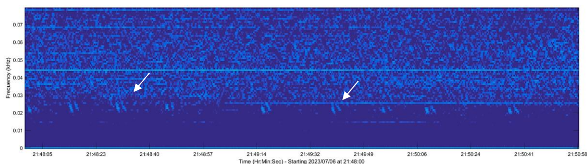
Figure 53 : « 20-Hz signal » émis en doublet par un Rorqual commun, Balaenoptera physalus , à proximité de la station R3. Enregistrement du 06/07/2023 vers 21h48 UTC.
