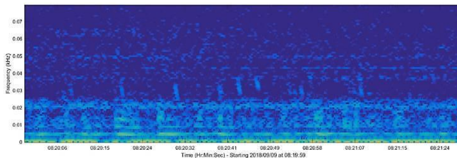
Figure 32 : Pulses (« down sweep ») émis par un Rorqual commun ( Balaenoptera physalus ) entre 20 et 40 Hz. Source : Quiet-Oceans, enregistrement recueilli le 09/09/2018 via un hydrophone positionné à 35m de profondeur en mer Méditerranée.
