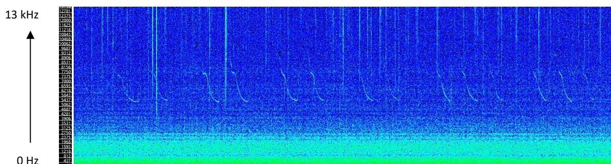
Figure 45 : Sifflements émis par le Grand Dauphin ( Tursiops truncatus ) entre 5 et 10 kHz le 07/03/2023 vers 09h06 UTC au niveau de la station R1.
