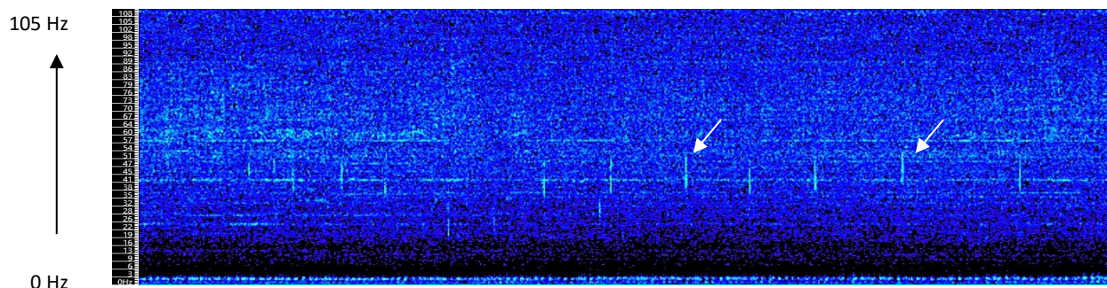
Figure 44 : Pulses émis par le Rorqual commun, Balaenoptera physalus , entre 55Hz et 38 Hz (« downsweep chirp ») à proximité de la station R3. Enregistrement du 15/03/2023 vers 04h00 UTC.
