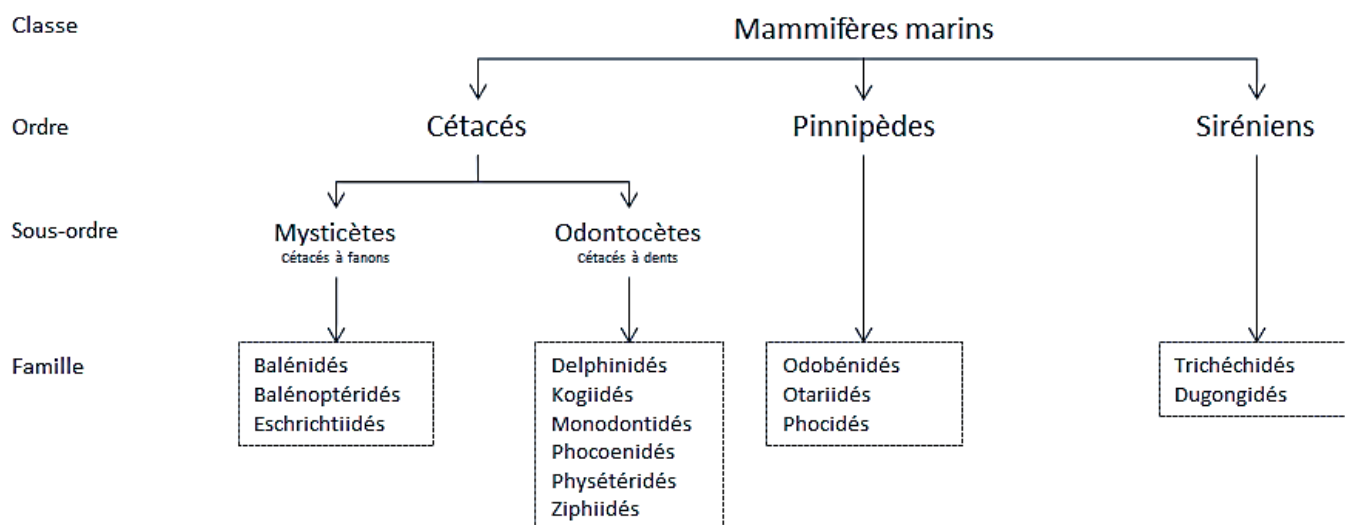
Figure 25 : Schéma de la classification scientifique des espèces océaniques et marines de mammifères. Source : Quiet-Oceans.
