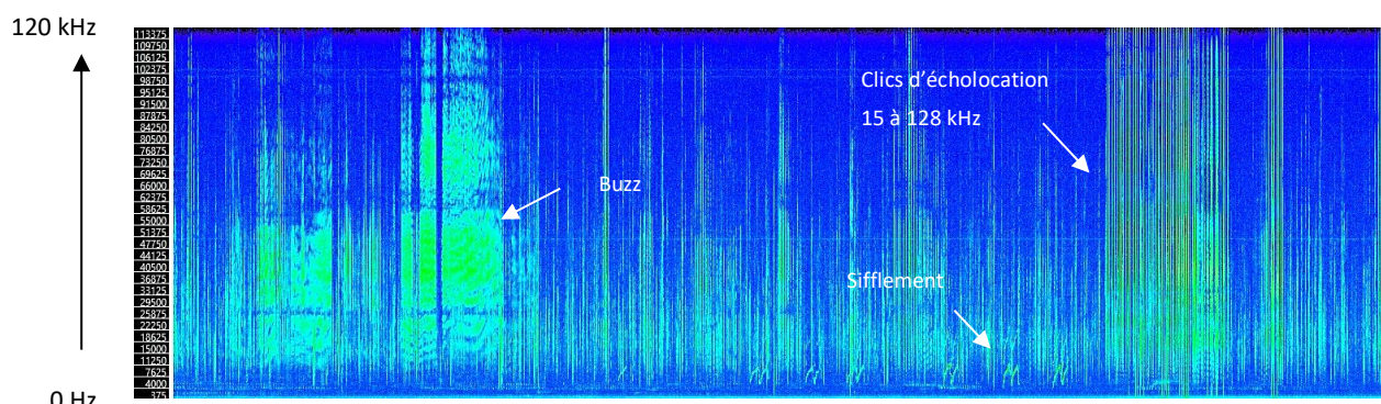
Figure 48 : Episode de communication intense évoquant une quête de nourriture par les Delphinidés au niveau de la station R1. Enregistrement du 08/07/2023 vers 11h21 UTC.
