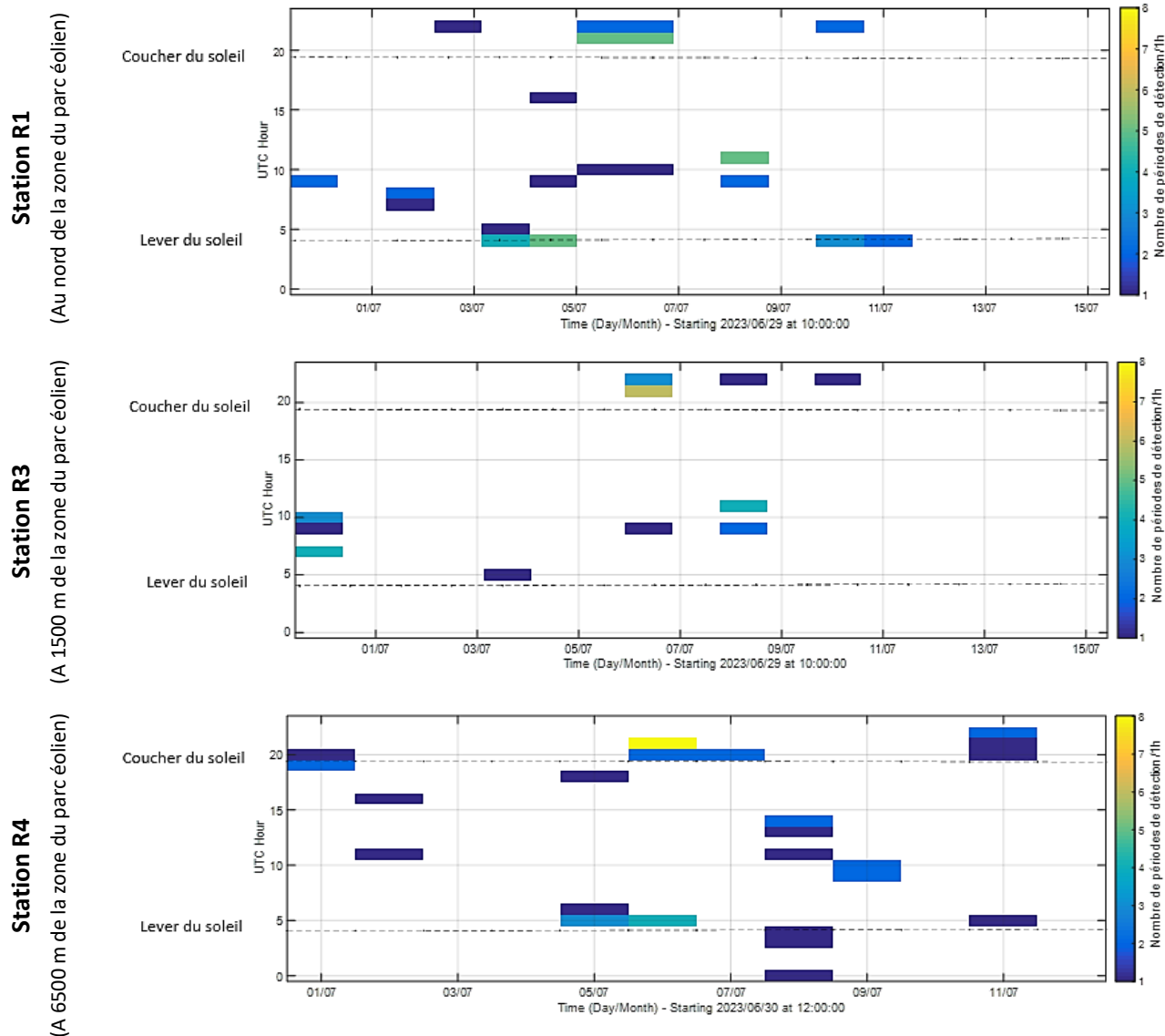
Figure 47 : Périodes de détections des clics et sifflements de Delphinidés en fonction du jour et de la nuit au niveau de chaque station (R1, R3 et R4) entre le 29 juin et 15 juillet 2023.
