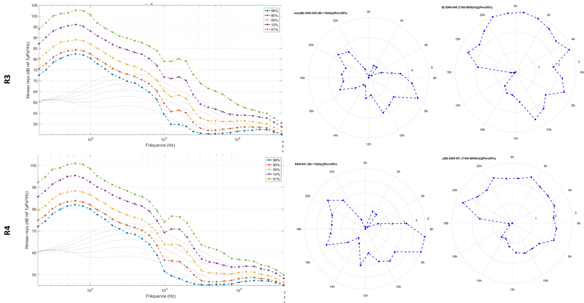
Figure 12 : Répartition fréquentielle de l'énergie acoustique mesurée en hiver/printemps 2023 (à gauche). Répartition horaire des émergences sonores en hiver/printemps 2023, au percentile 50% dans les bandes 89Hz-110Hz (au centre) et 7.1-8.9kHz (à droite).
