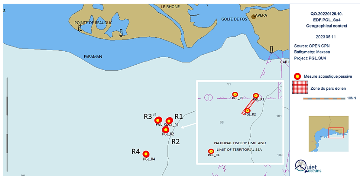
Figure 6 : Protocole géographique des mesures longues durées.
