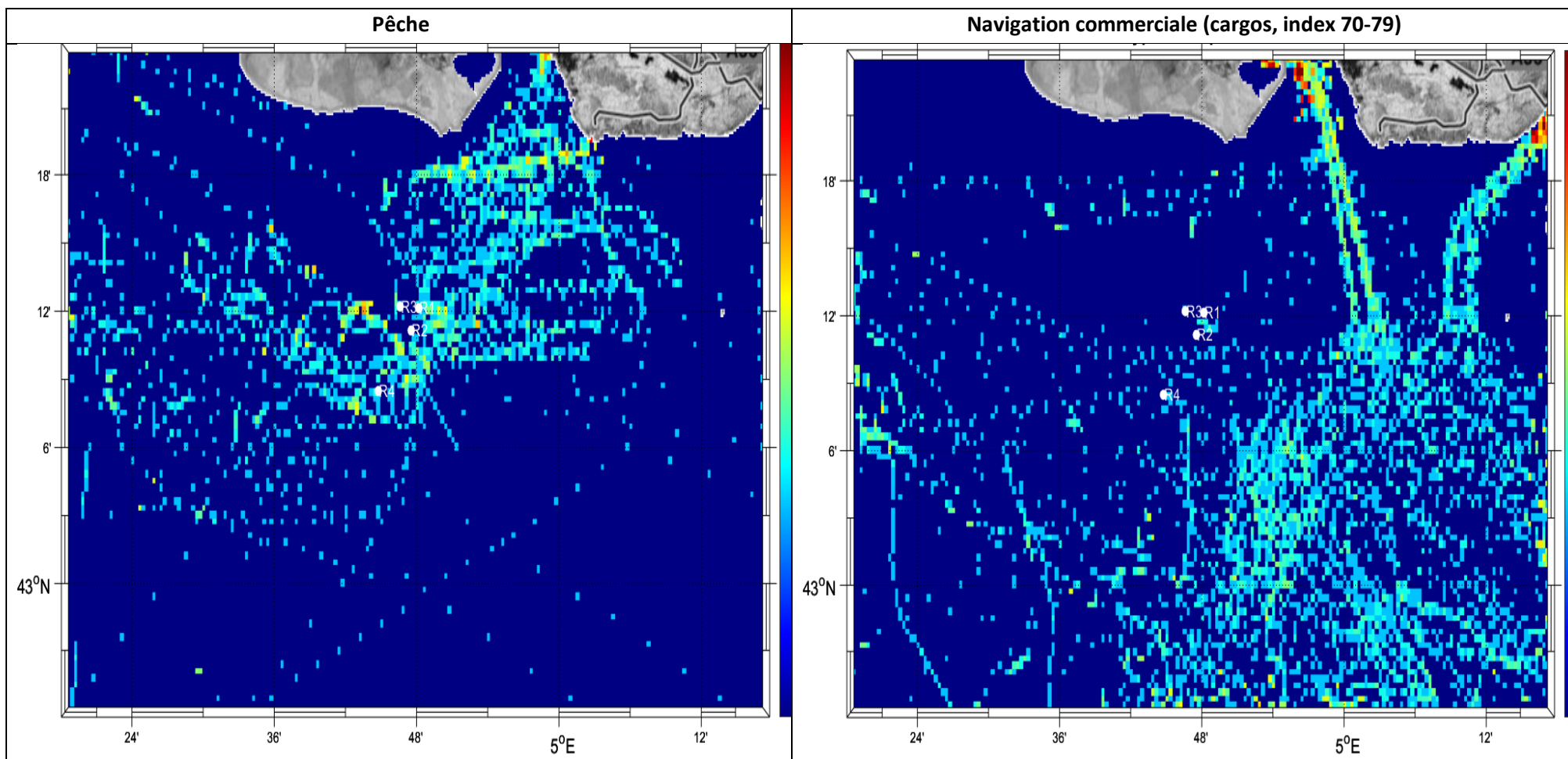
Figure 21 : Densité de trafic dans la zone au mois de Mars 2023.
