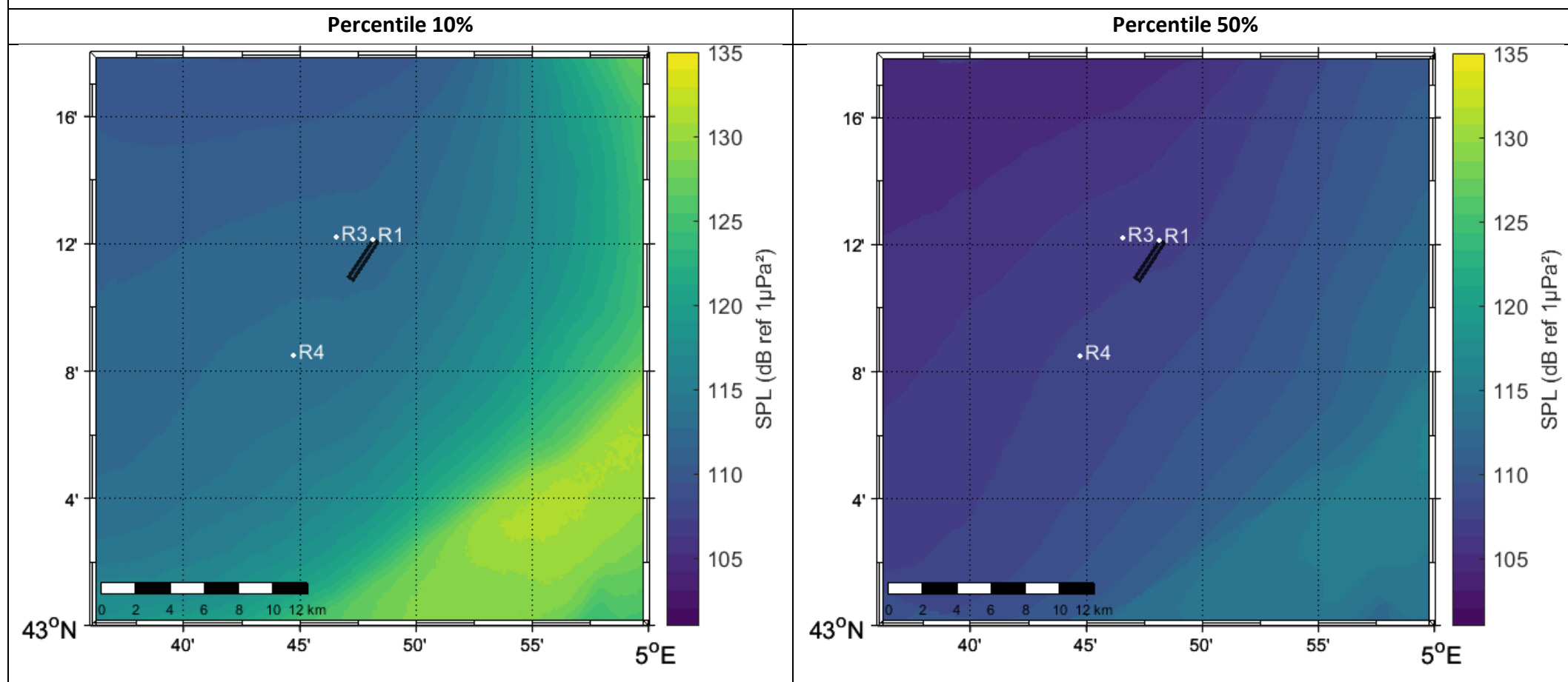
Figure 24 : Cartographie statistique du bruit (entre 20 Hz et 5.65 kHz) par mois, calculée aux percentiles 10% (à gauche) et 50% (à droite).
