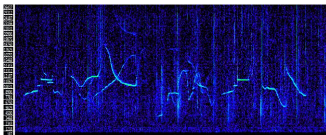
Figure 30 : Sifflements de Delphinidés émis entre 2 kHz et 25 kHz. Source : Quiet-Oceans.
