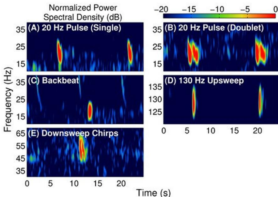
Figure 33 : Pulses émis par le Rorqual commun ( Balaenoptera physalus ).
