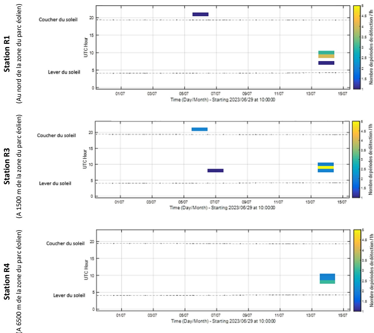
Figure 51 : Périodes de détections des pulses émis par les Rorquals communs ( Balaenoptera physalus ) en fonction du jour et de la nuit au niveau de chaque station (R1, R3 et R4) entre le 29 juin et 15 juillet 2023.
