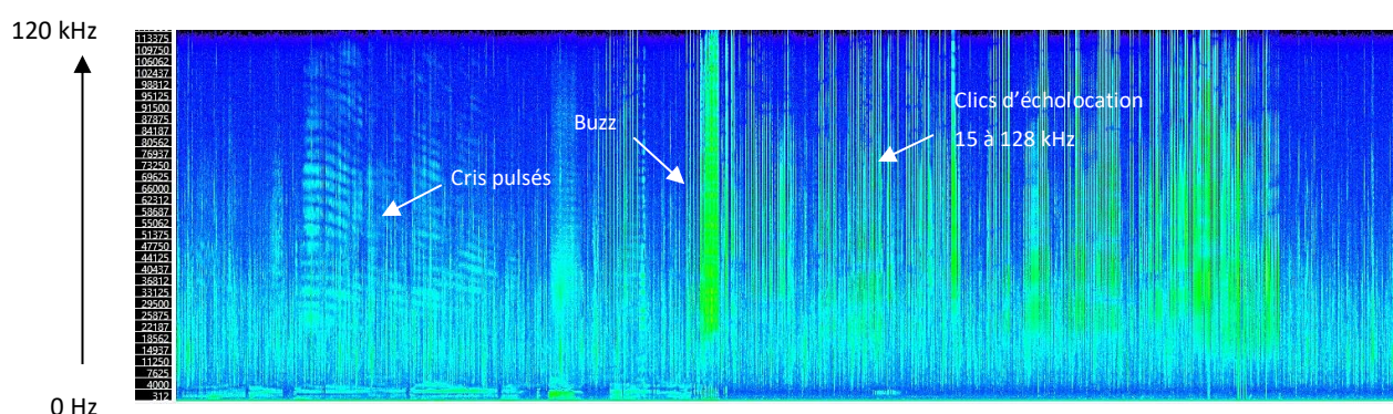
Figure 50 : Episode de chasse opportuniste observé lors de l'analyse bioacoustique des résultats concernant les Delphinidés à proximité de la station R4. Enregistrement du 06/07/2023 vers 21h55 UTC.
