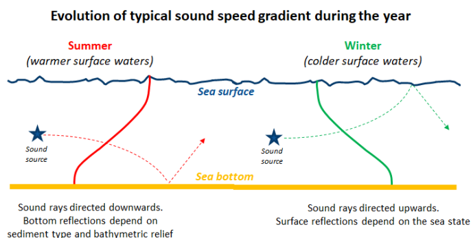
Figure 5 : Illustration schématique des effets de la variation du profil de célérité sur la propagation du son (source Quiet-Oceans)
