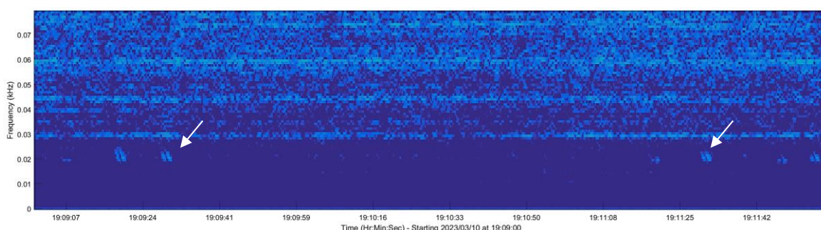
Figure 43 : Pulses émis en doublet par un Rorqual commun, Balaenoptera physalus , entre 27 Hz et 17 Hz (« 20-Hz signal ») à proximité de la station R4. Enregistrement du 10/03/2023 vers 19h09 UTC.
