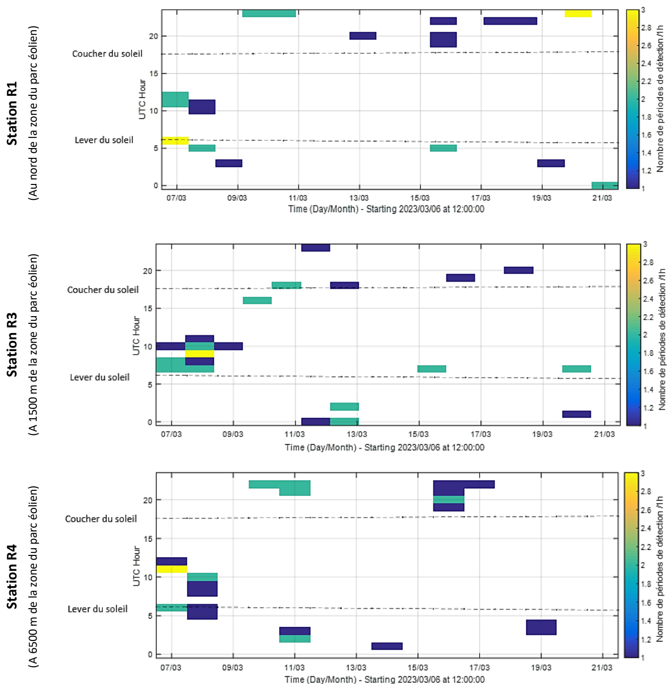
Figure 36 : Périodes de détections des clics et sifflements de Delphinidés en fonction du jour et de la nuit au niveau de chaque station (R1, R3 et R4) entre le 06 et 21 mars 2023.
