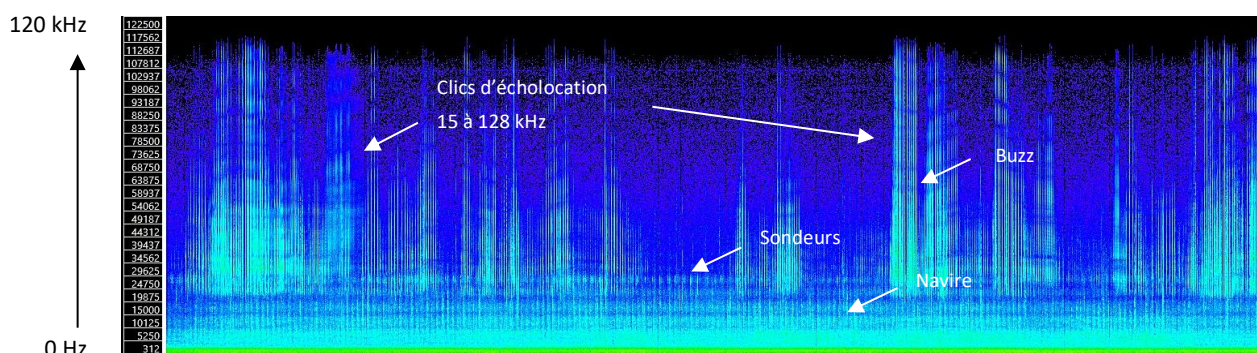
Figure 38 : Trains de clics d'écholocation et buzz émis par les Delphinidés entre 15 et 128 kHz à proximité de la station R3. Enregistrement du 15/03/2023 vers 06h19 UTC.
