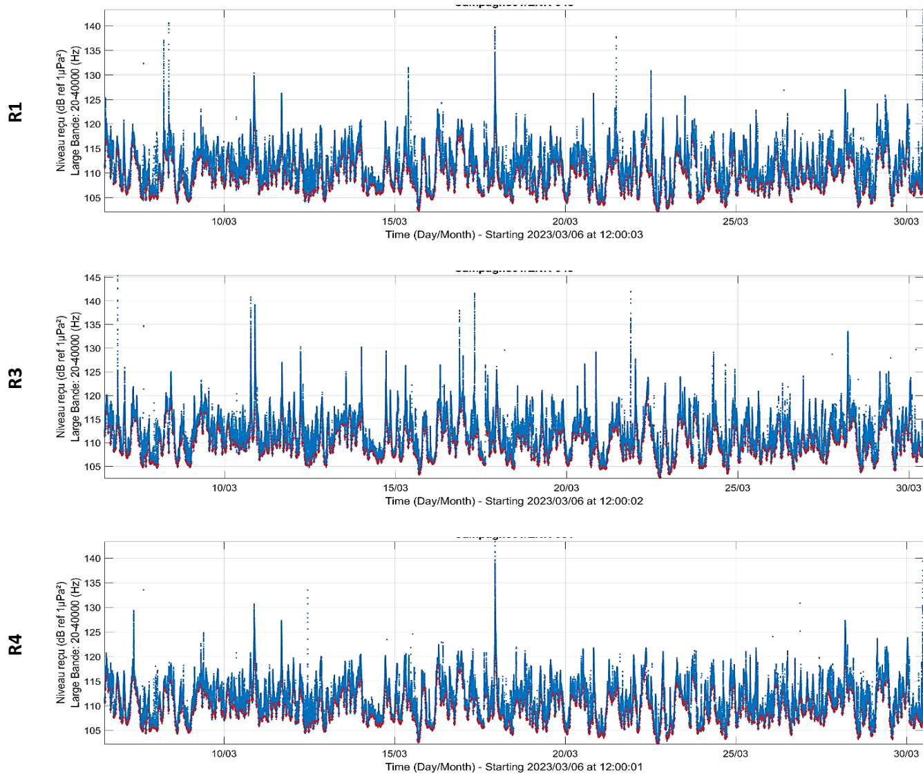
Figure 8 : Evolution des niveaux intégrés dans la bande [20Hz;40kHz] (exprimés en dB ref 1µPa²) mesurés lors de la période hiver/printemps 2023.
