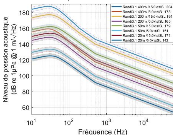
Figure 22 : Gabarit sonore des navires en fonction de la longueur, la vitesse et la fréquence
