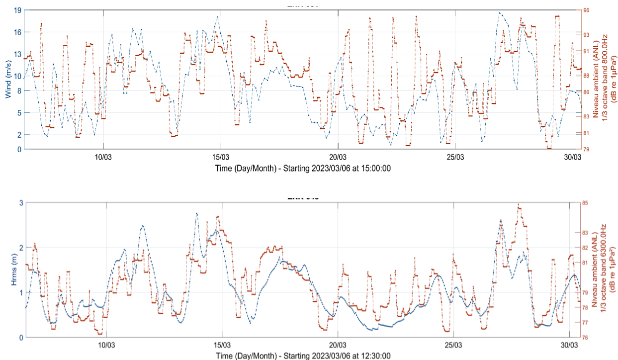
Figure 9 : Corrélation du bruit permanent (orange) avec les conditions météorologiques (bleu) dans la zone d'étude lors de la période hiver/printemps 2023.
