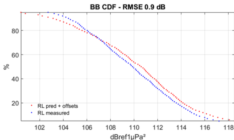
Figure 23 : Distribution des niveaux sonores (en rouge, courbe prédite, en bleu, donnée mesurée) à la station R1, à l'issue du processus de calibration.
