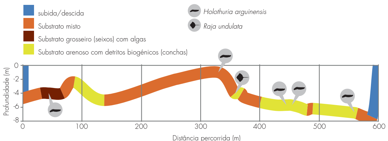
Figura 8. Perfil do transecto realizado pelo Veículo de Operação Remota (ROV), com o tipo de substrato e a fauna presente.
