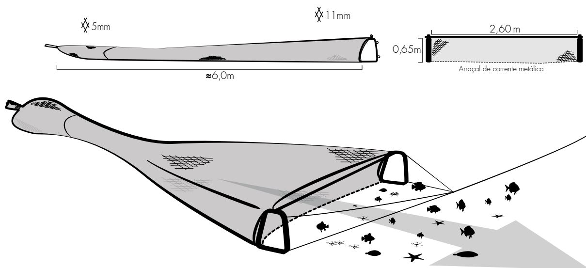
Figura 4. Detalhes e modo típico de operação da arte de pesca utilizada para amostragem das comunidades de substratos móveis.
